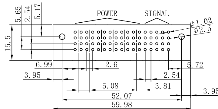
P.C.Body Hole Layout
